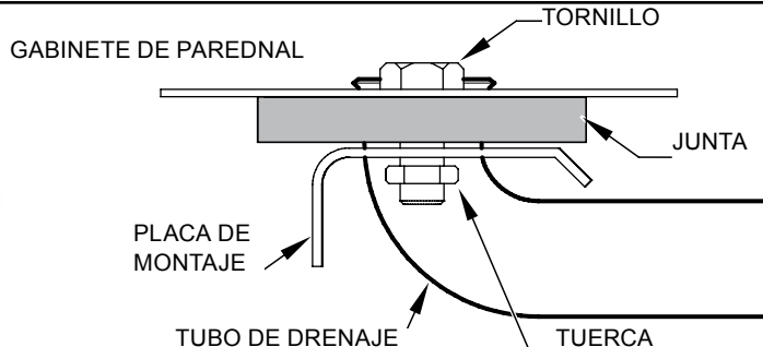
VISTA LATERAL
