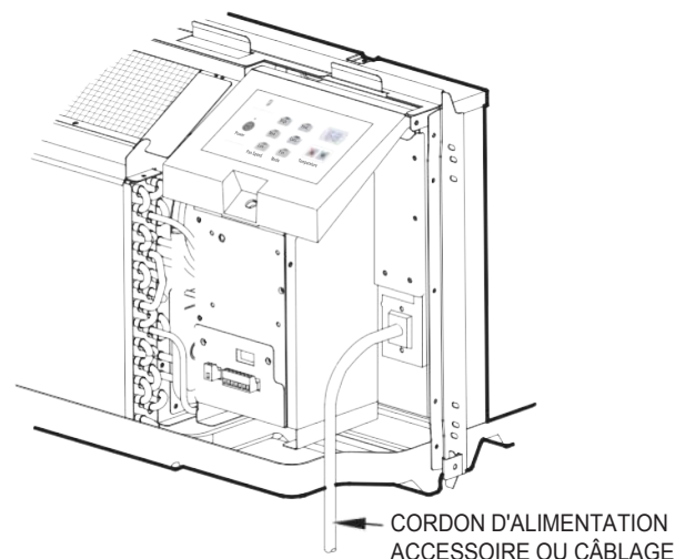
Figure 26 Connexion de l'alimentation
