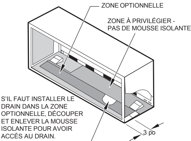
Figure 11 Emplacement et installation du nécessaire de drainage
