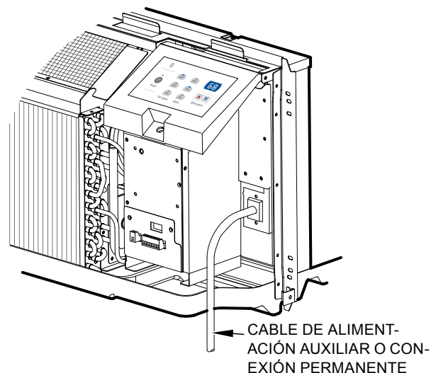
Figura 26 Conexión Eléctrica
